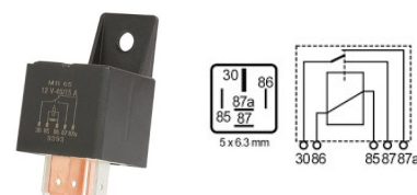
MR65/RELÉS-C/RESISTENCIA
