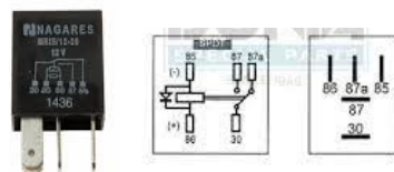
MR3/MICRORELÉS
