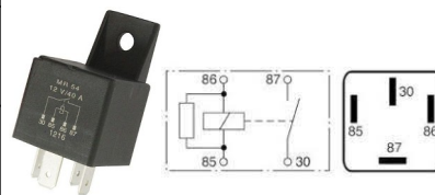
MR56/RELÉS-C/RESISTENCIA
