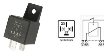
MR54/RELÉS
